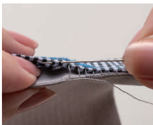
10 用包邊縫合封口返口。
